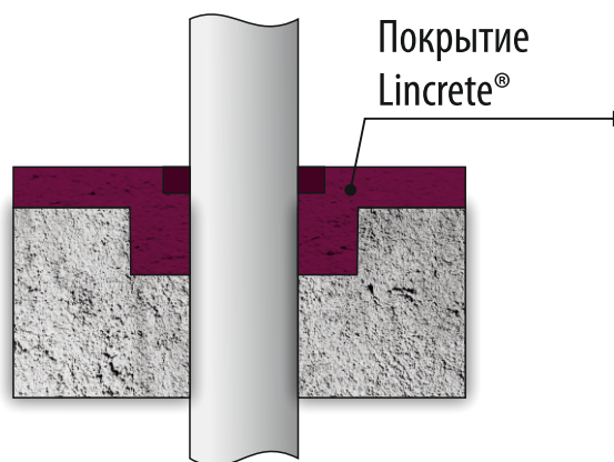
Примыкание к сквозным коммуникациям
